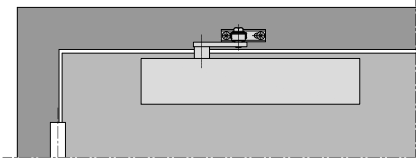
1.1 Scherenarmschließer Türblattmontage Bandseite (Türblatt stumpf)
