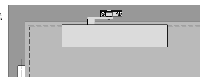
1.2 Scherenarmschließer Türblattmontage Bandseite (Türblatt gefälzt)
