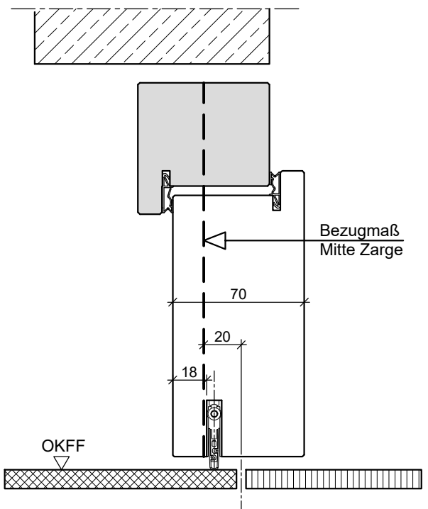
HR70-gefälzt
