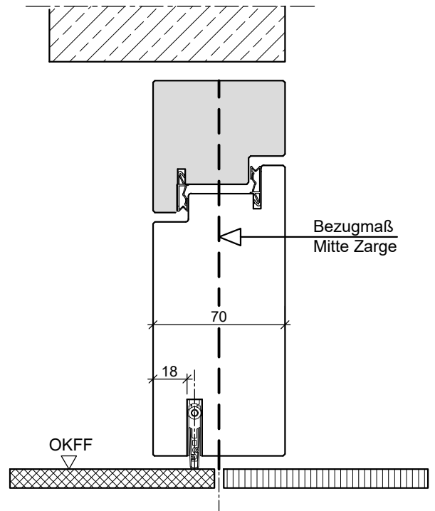
HR70-Doppelfalz
