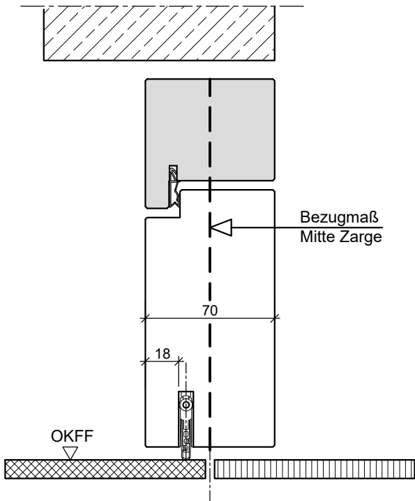
HR70-flächenbündig
